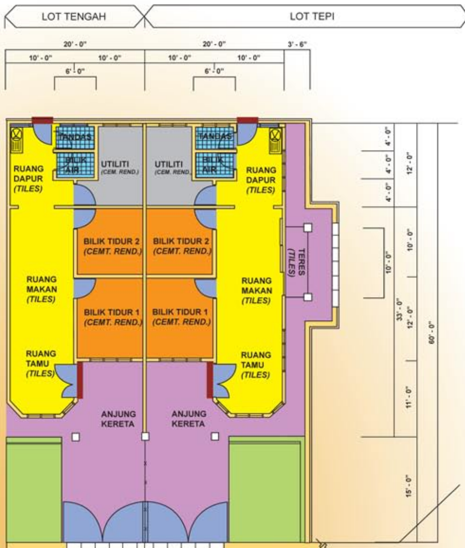
PELAN LANTAI Tanpa Skala
